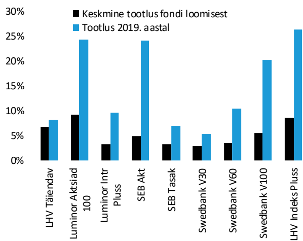
Joonis 38. III samba fondide tootlused fondi loomisest 9 ja 2019. aastal.
