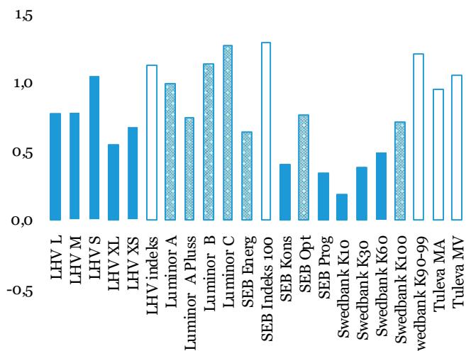
Joonis 20. II samba fondide Sharpe'i suhtarv*
